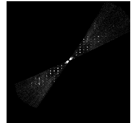
Etude de la diffusion diffuse et du désordre dans ZSM-48
