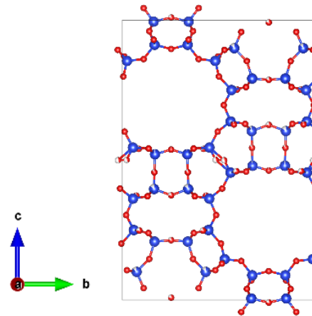
Localisation de cations dans ECR-1
