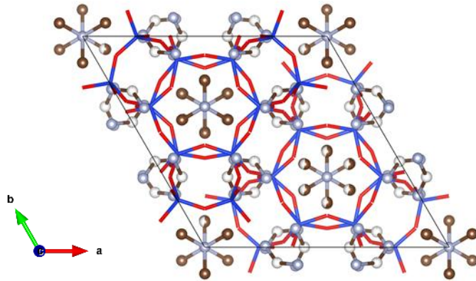
Localisation de l'agent structurant dans CHA
