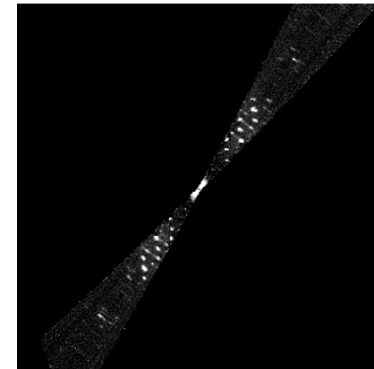
Etude de la diffusion diffuse et du désordre dans ZSM-48
